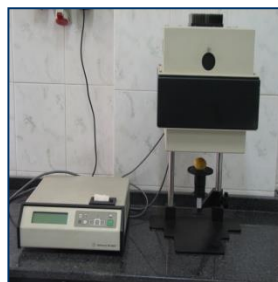
دستگاه رنگ سنج هانتر لب
