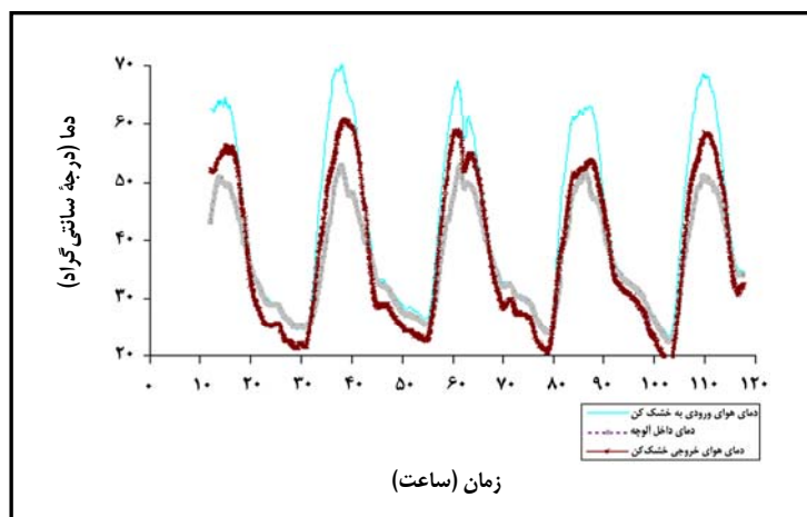
شکل ۲- تغییرات دمای خشک کن و میوه طی خشک شدن آلوجه در خشک کن آفتابی
