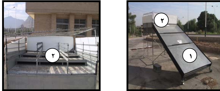
شکل ۱- خشک کن آفتابی و قسمت های آن (۱- جمع کننده حرارتی و ۲- اتاقک خشک کن)
