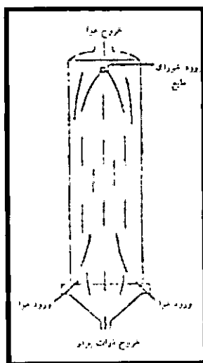
شکل ۷- خشک‌کن پاششی جریان غیر هم‌سو
