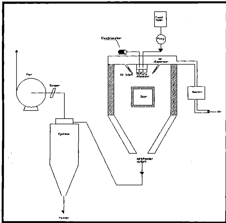
شکل ۱- خشک کن پاششی و اجزاء آن
