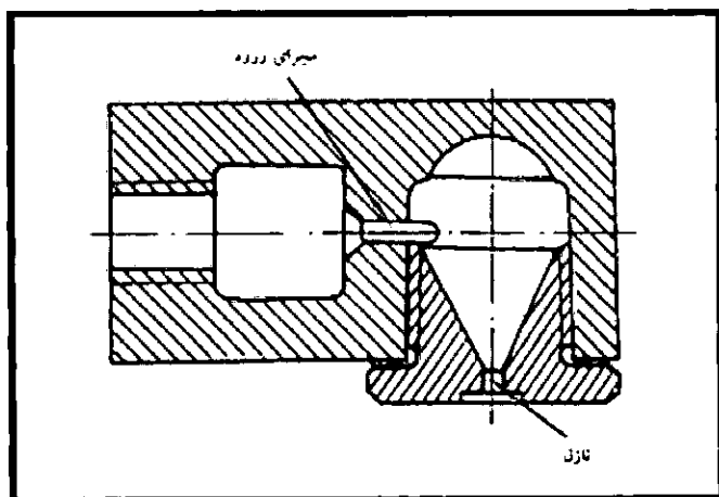
شکل ۴- افشانک فشاری
