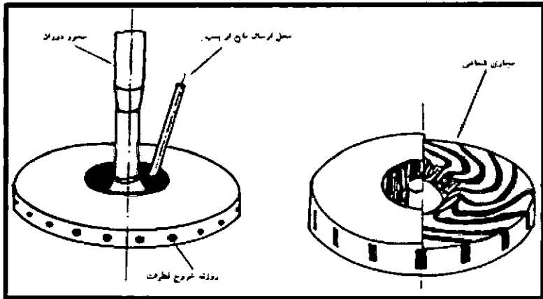
شکل ۲- قسمت‌های مختلف یک افشانک چرخ دوار
