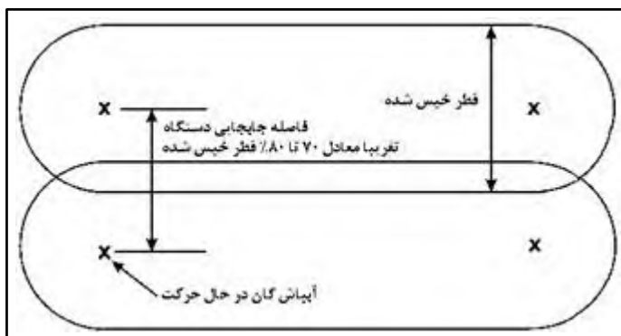
شکل ۷- فاصله جابجایی دستگاه یا فاصله بین دو مسیر حرکت آبیاش
