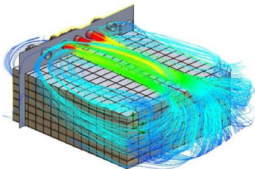
شکل ۴- شبیه‌سازی رایانه‌ای، آگاهی ما را از وضعیت جریان هوا در انبارهای نگهداری افزایش داده است
