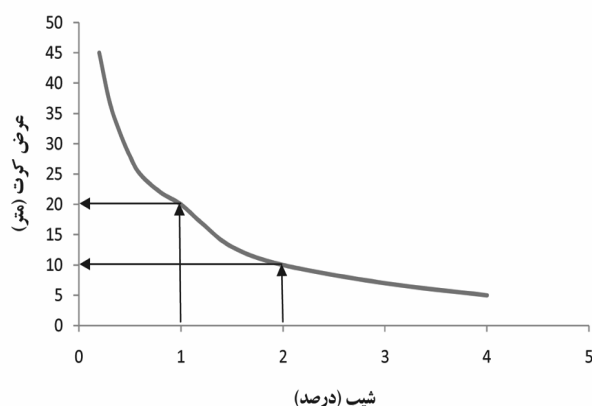
شکل ۳۱- عرض کرت در آبیاری کرتی به صورت تابعی از شیب مزرعه
