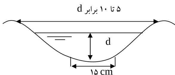
شکل ۴۲- نمایی از شکل شیار در یک خاک رسی در آبیاری شیری (عریض و کم عمق، d عمق آب داخل شیار است)
