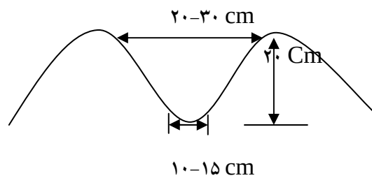
شکل ۴۱- نمایی از شکل شیار در یک خاک شنی (عمیق و باریک)
