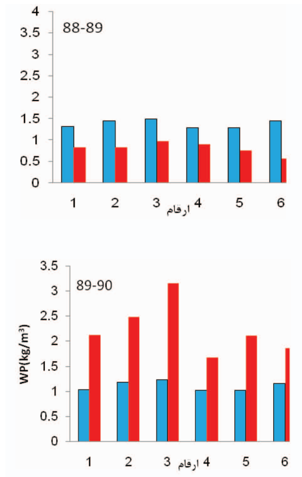
شکل ۶۴- بهره‌وری آب ارقام مختلف گندم به تفکیک چهار سال ( ستون آبی و قرمز به ترتیب نماینده‌ی بهره‌وری بارش و آب آبیاری است)
