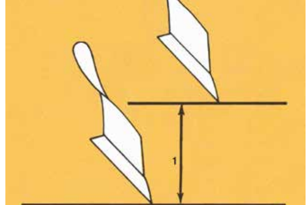
Fore-and-Aft clearance فاصله نوک یک تیغه تا نوک تیغه بعدی (در گاوآهن برگردان دار)
