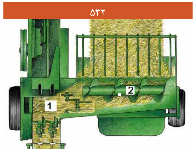
1-Bale chamber 2- Auger ۱-محفظه بسته بندی ۲-مارپیچ
