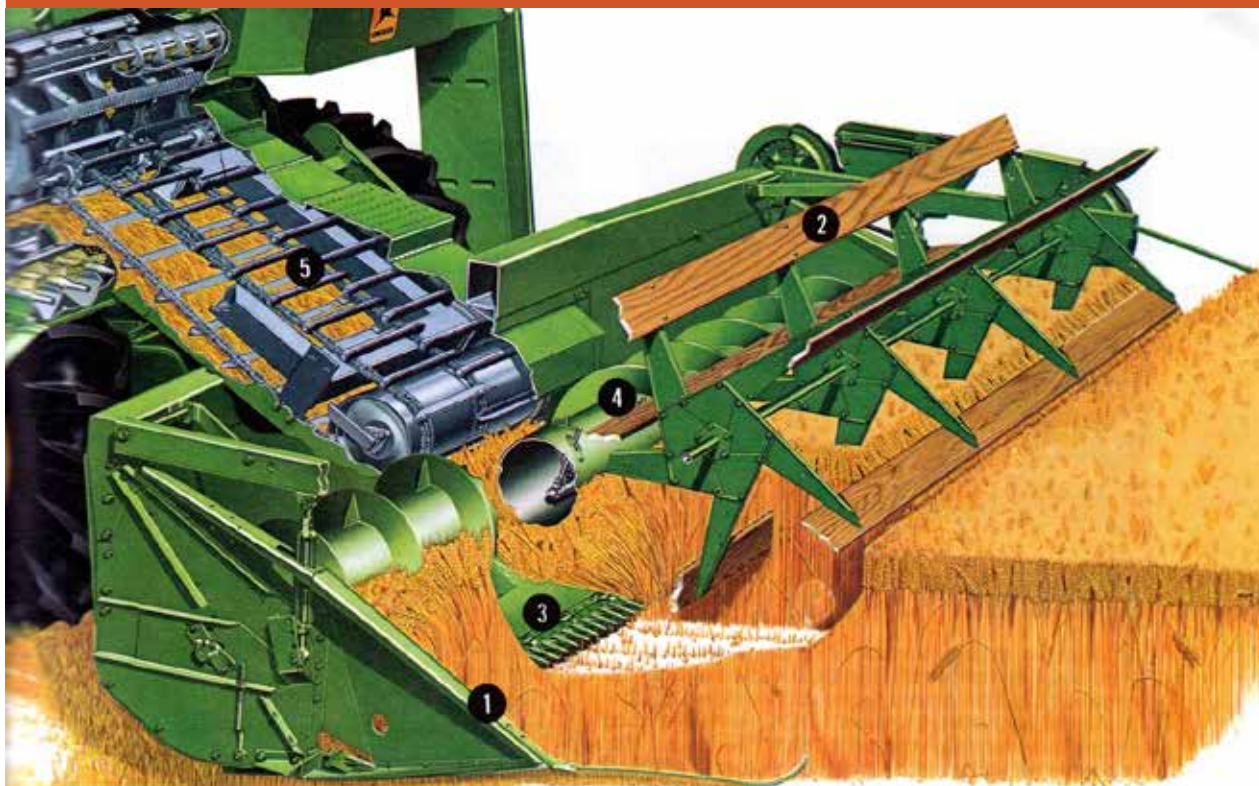
1-Divider 2-Slat reel 3-Cutter bar 4-Auger 5-Feeding conveyor ۱- تقسیم‌کننده ۲- چرخ فلک پره‌ای ۳- شانه برش ۴- ماریج ۵- نقاله تغذیه
