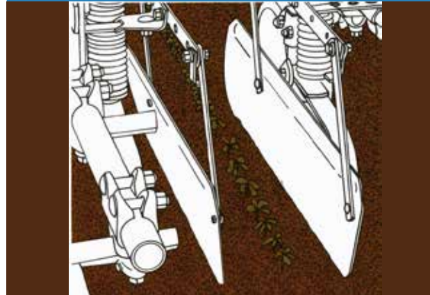
Rig attached cultivator plant shields کلتیواتور دارای محافظ گیاه
