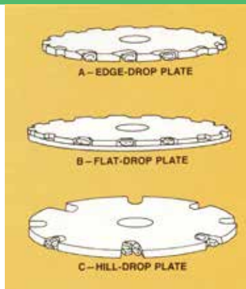
1-Edge drop plate 2-Flat-drop plate 3-Hill drop plate ۱-صفحه کنار ریز ۲-صفحه مسطح ریز ۳-صفحه کپه ریز
