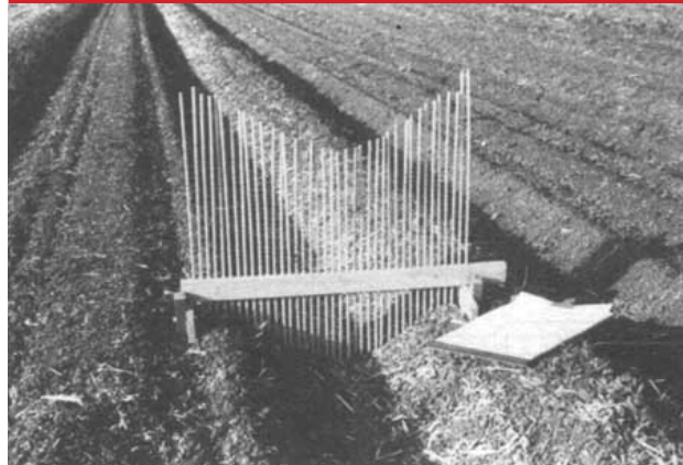
Furrow cross section مقطع شیار ضخیم
