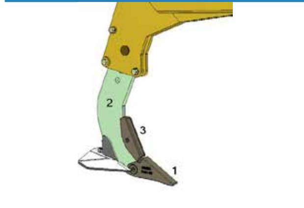
1-point 2- Standard 3- Shin ۱- تیغه (نوک) ۲- ساقه = دسته = دستک = پایه ۳- پیشانی
