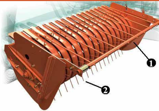
1-Compressor 2- Pickup ۱- فشرده ساز ۲- بردارنده علوفه
