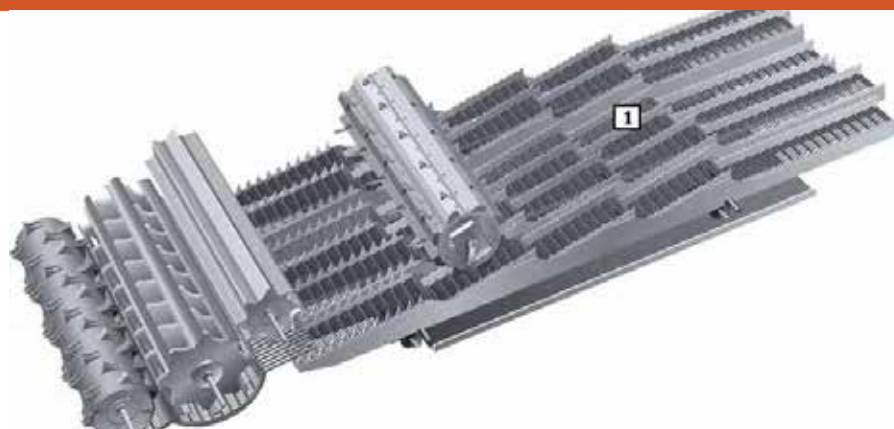
1-Separating unit ۱- واحد جدا کننده
