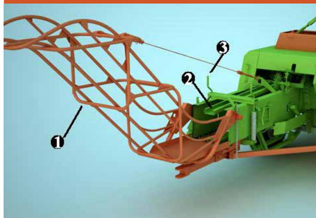
1- Bale chute 2- Tension bar 3- Tension crank ۱- شوت بسته ۲- میله فشرده کننده بسته ۳- دسته فشار = هندل فشار
