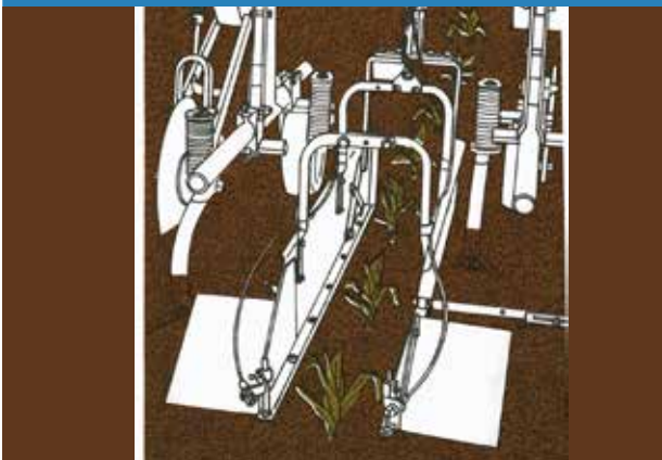
Spray cultivator shields محافظ سمپاش کلتیواتور
