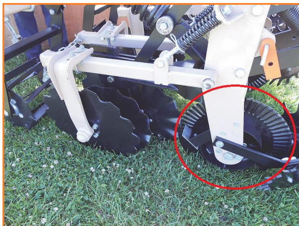
شکل ۲۲- پیش‌بر بشقابی شیاردار
