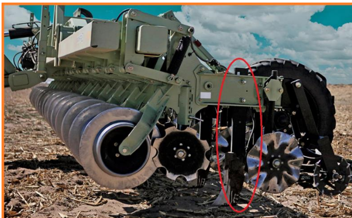
شکل ۳۰- ساق زیرشکن
