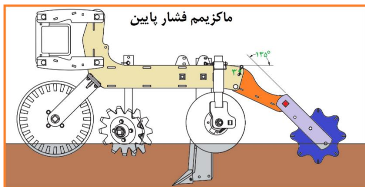
شکل ۷۶- اتصال در نقطه ۳ برای ماکزیمم فشار پایین (منبع: بیگ هام، ۲۰۲۱)
