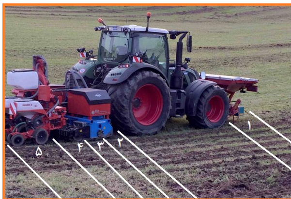
شکل ۷۹- ماشین مرکب با ترکیب ماشین کودپاشی، خاک‌ورز نواری فعال و ماشین کاشت
