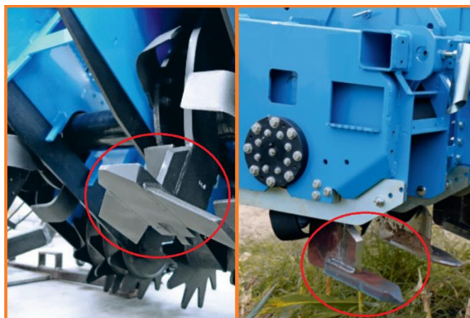
شکل ۸۱- شاخه زیرشکن
