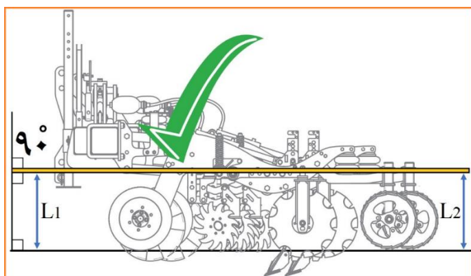
شکل ۵۶- برقرار بودن تراز طولی (منبع: اس ال وای فرانسه، ۲۰۱۵)
