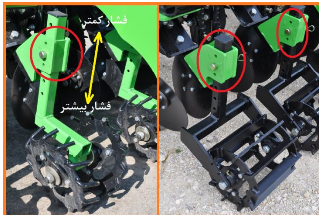
شکل ۷۰- تنظیم جابجایی شاسی غلتک روی شاسی ماشین
