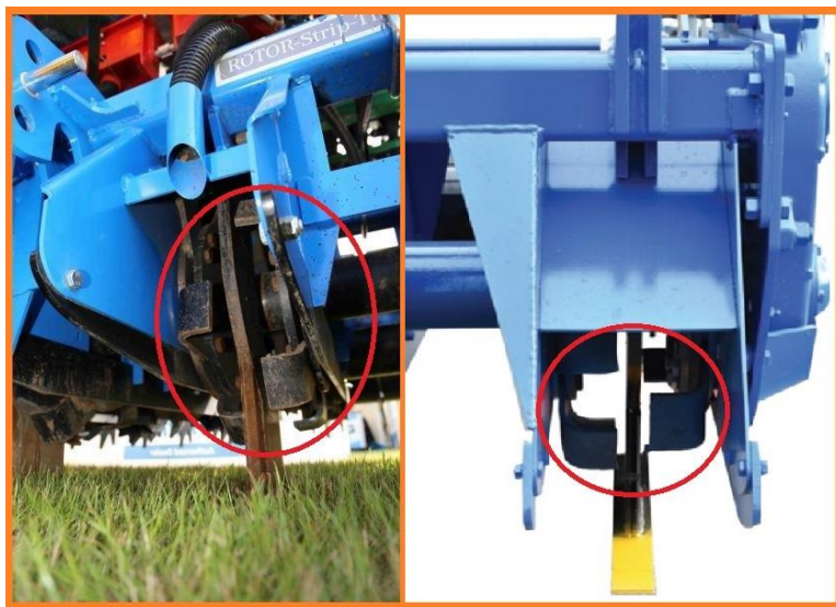
شکل ۸۴- تیغه‌های L شکل
