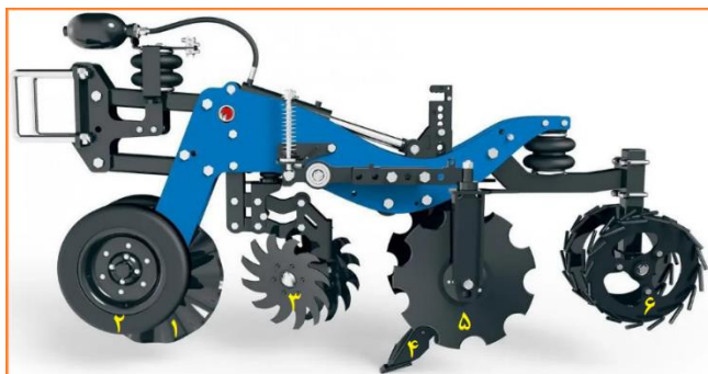
شکل ۸- ماشین خاک‌ورز نواری غیرفعال (۱- پیش‌بر بشقابی ۲- چرخ کنترل عمق ۳- ردیف ساز بشقابی ۴- ساق زیرشکن ۵- خردکن بشقابی ۶- کلوخ خردکن)
