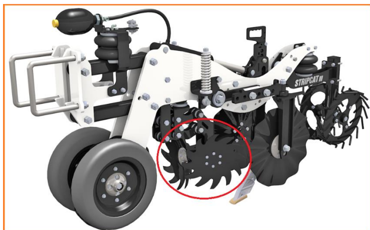
شکل ۲۶- ردیف ساز چرخ انگشتی دار
