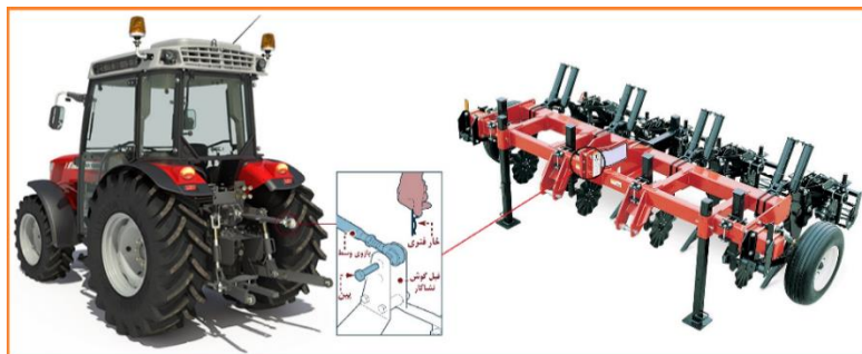
شکل ۵۲- اتصال بازوی وسط تراکتور به ماشین
