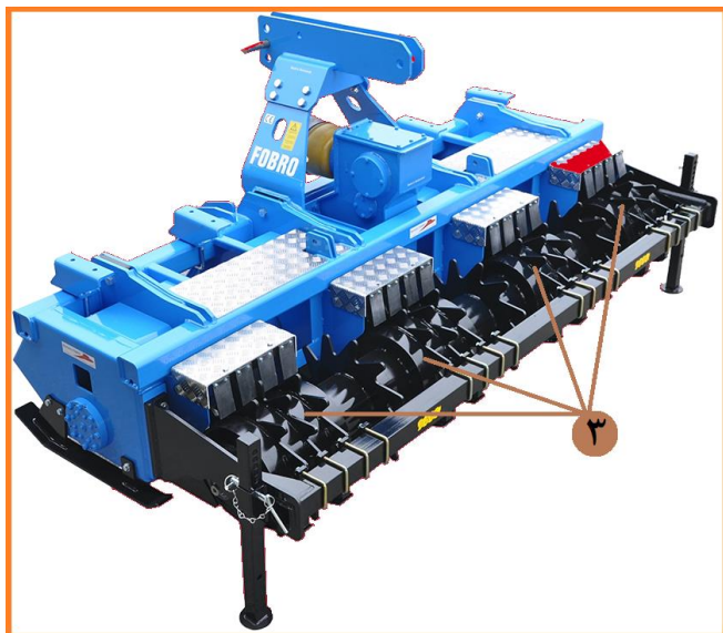
شکل ۱۰- ماشین خاک‌ورز نواری فعال (از عقب) (۳-غلتک با زائده کاردی)
