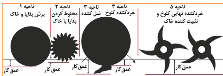
شکل ۱۵- اجزای درگیر با خاک در ماشین خاک‌ورز نواری غیرفعال (منبع: فارمت، ۲۰۲۱)
