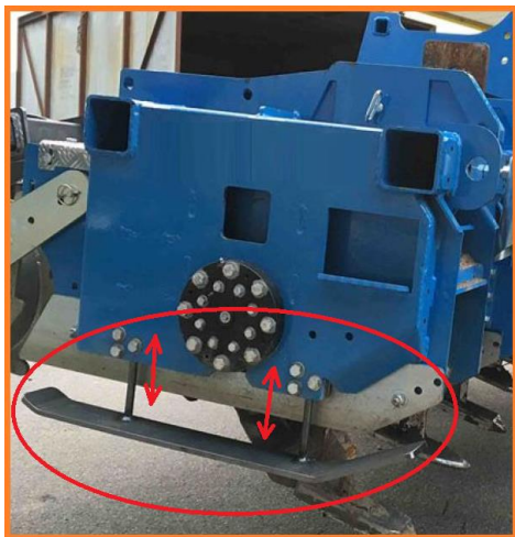
شکل ۸۸- کفشک‌های تنظیم عمق
