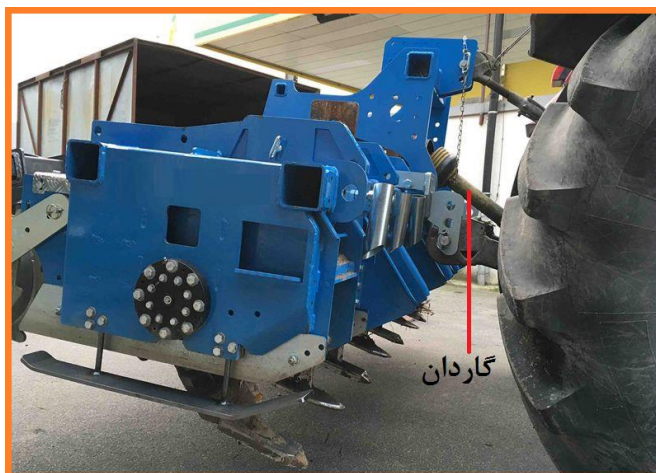
شکل ۱۱- انتقال قدرت دورانی از محور توان‌دهی تراکتور
