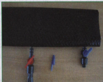
شیر انشعاب تیپ، لوله پنج لایه نخدار و لوله تیپ
