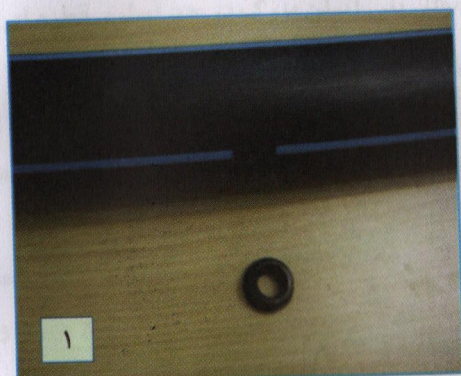
شکل ۱۱- نحوه انشعاب آب از لوله آب رسان پلی اتیلن ۶۳ میلی متری با واشر به لوله تیپ با انشعاب شیردار
