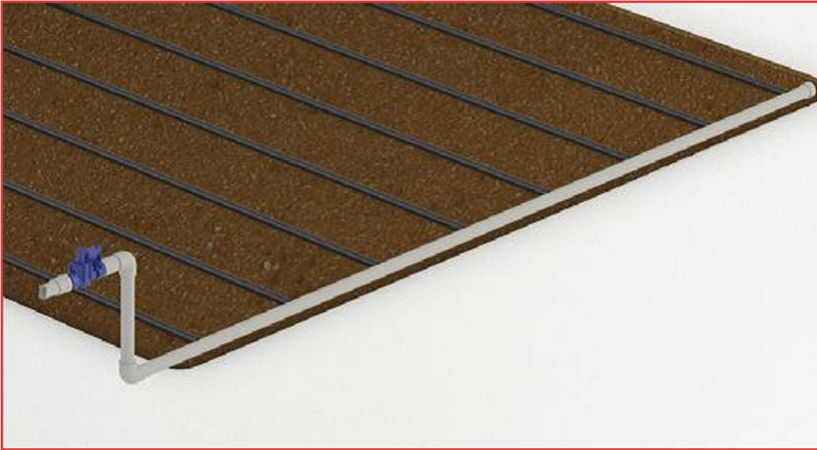
شکل ۱۲- شماتیک مانیفولد شست‌وشو در آبیاری قطره‌ای
