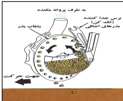
شکل ۱۰- موزع صفحه‌ای تحت مکش در ردیف کار پنوماتیکی برای کاشت بادام زمینی
